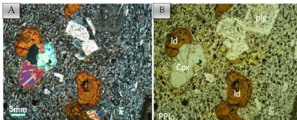
شکل ۱۲. تصاویر میکروسکوپی یک نمونه بازالت پورفیری از منطقه قم. بلورهای اولیون کم و بیش ایدنگسیستی شده‌اند. (A) با آنالیزور، (B) بدون آنالیزور
