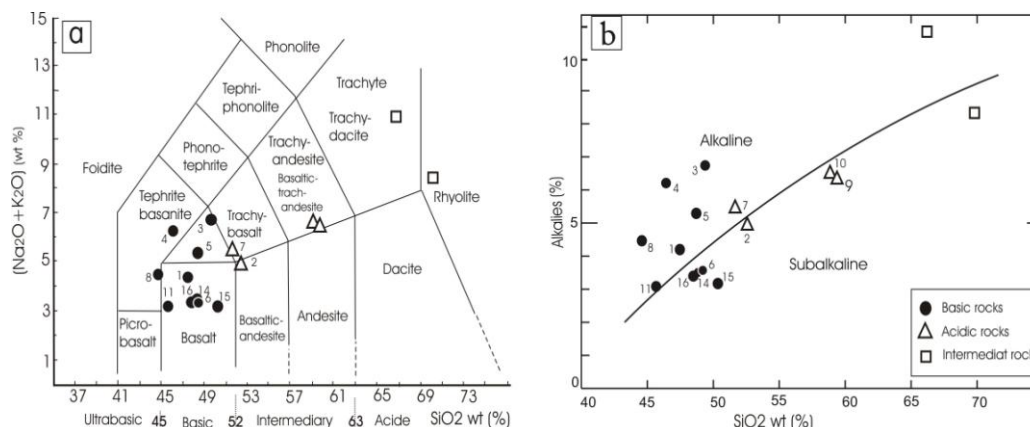
شکل ۹. موقعیت نمونه‌های سنگ‌های آتشفشانی منطقه در طبقه‌بندی [۸] و در نمودار آلكالین- سیلیس [۹]
