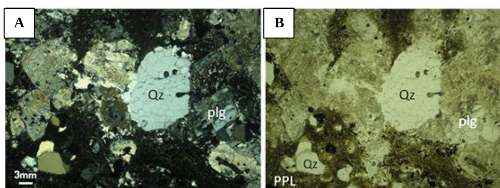
شکل ۱۵. یک نمونه ریولیت متشکل از کوارتز، لاژیوکلاز سدیک و خمیره‌ای فلسیتیک. (A) در آنالیزور، (B) بدون آنالیزور
