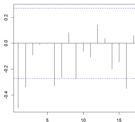
شکل ۳. نمودار pacf مقادیر تفاضل‌گیری شده
