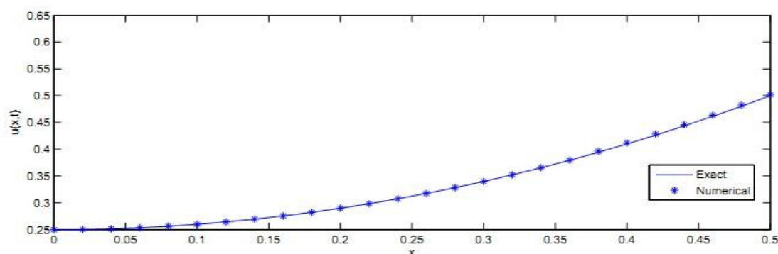
شکل ۵. مقایسه جواب دقیق با جواب به دست آمده از طرح تفاضلات متناهی غیر استاندارد به ازای m=25 در t=0.5
