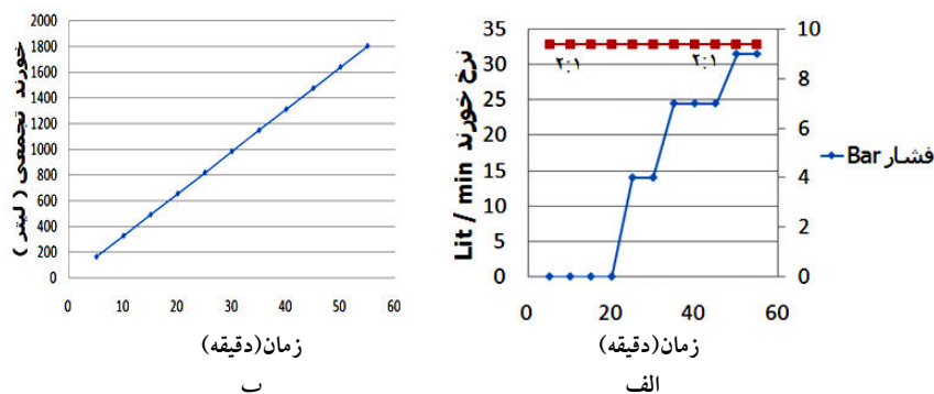
شکل ۷. الف) نمودار نرخ خوردند- زمان - فشار مقطع ۷۰-۸۰ از گمانه (PR29) ب) نمودار خوردند تجمعی- زمان مقطع ۷۰-۸۰ از گمانه (PR29)
