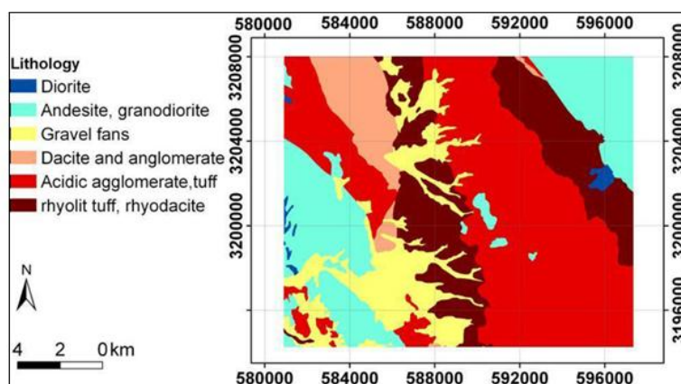
شکل ۶. نقشه لیتولوژی (اقتباس از نقشه زمین‌شناسی ۱:۱۰۰۰۰۰ سبزواران)؛ طبق راهنمای نقشه از بالا به پایین پتانسیل لغزش افزایش می‌یابد.
