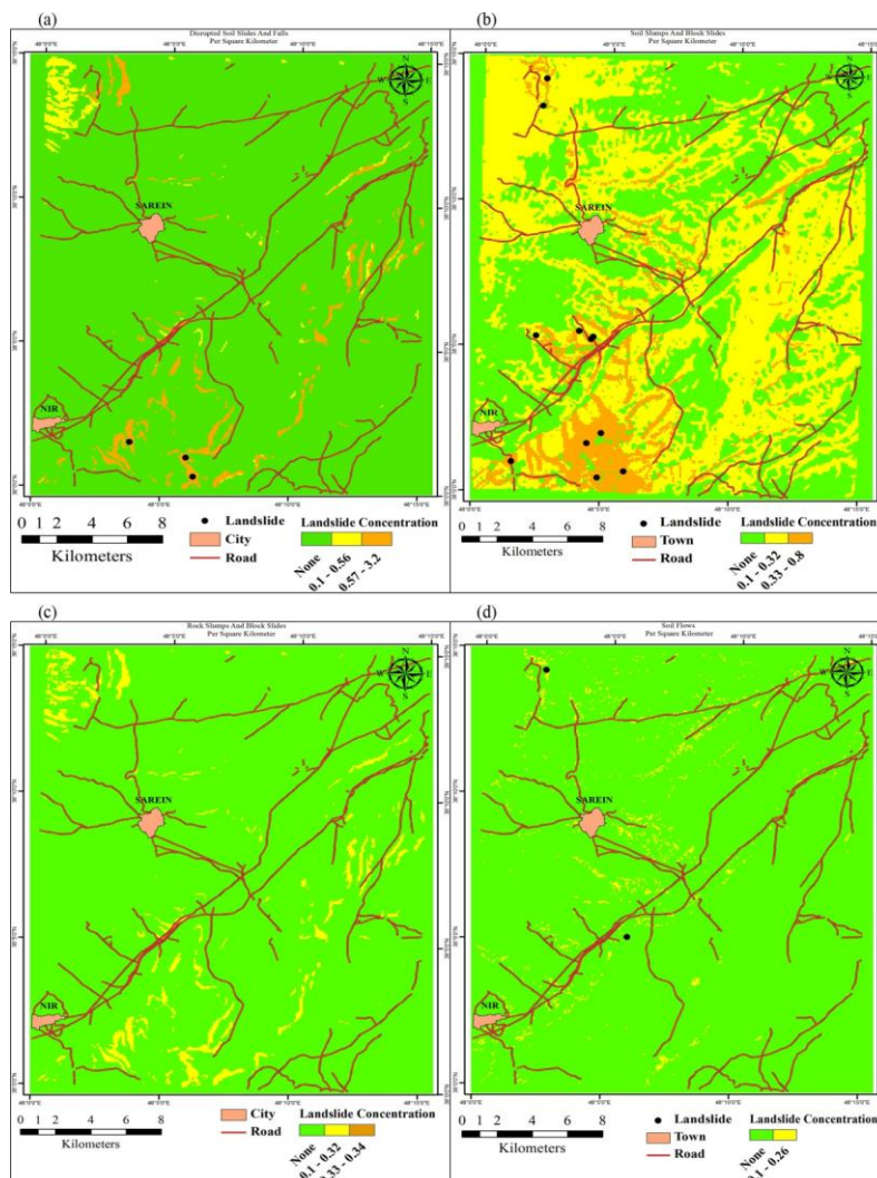
شکل ۱۲. تراکم خطر زمین‌لغزش‌های ناشی از زلزله محاسبه شده برای زلزله ۱۳۷۵ سرعین، اردبیل با M_w = 6.1 : (a) تراکم‌های پیش‌بینی شده ریزش‌ها و لغزش‌های خاکی گسسته با استفاده از کمل، (b) تراکم‌های پیش‌بینی شده لغزش‌های بلوکی و چرخشی خاکی با استفاده از کمل، (c) تراکم‌های پیش‌بینی شده لغزش‌های بلوکی و چرخشی سنگی با استفاده از کمل، (d) تراکم‌های پیش‌بینی شده جریان‌های خاکسریع با استفاده از کمل. دایره‌های توپر زمین‌لغزش‌های رخ داده ناشی از زلزله ۱۳۷۵ سرعین، اردبیل هستند.
