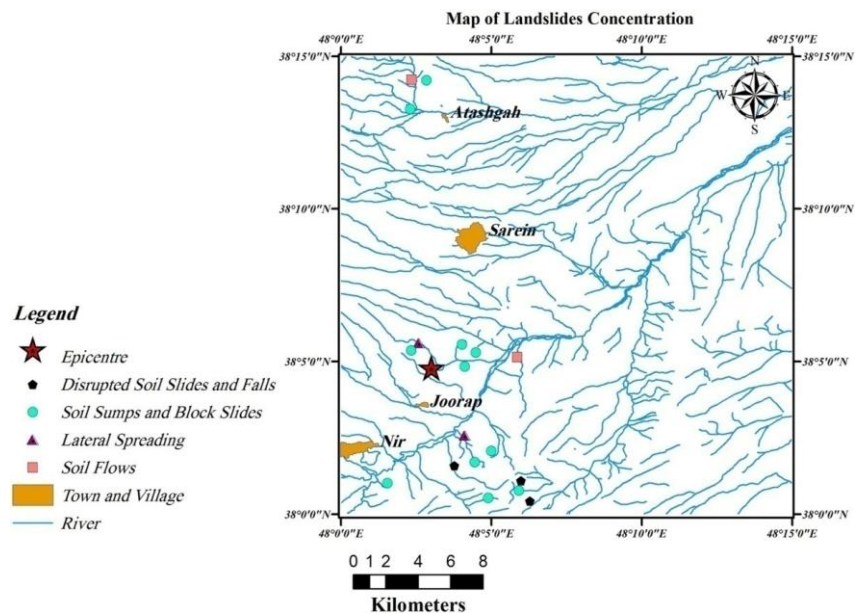
شکل ۳. نقشه پراکنش زمین‌لغزش‌های ناشی از زلزله ۱۳۷۵ سرعین در محدوده بررسی شده
