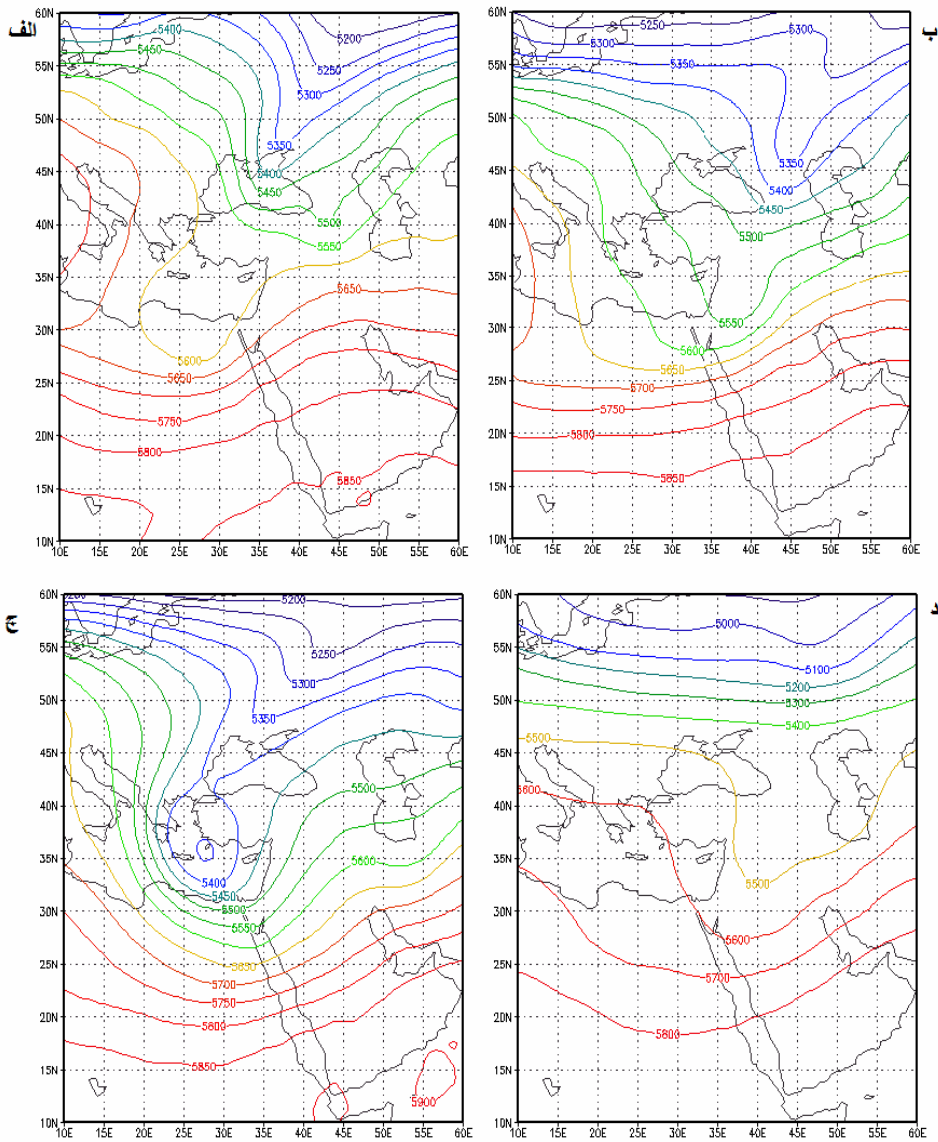
شکل (۱) مکان گزینی ناوه سامانه ترکیبی مدیترانه‌ای - سودانی در ساعات مختلف تراز ۵۰۰ هکتوپاسکال، (الف) ساعت 00 utc روز 4 فوریه ۱۹۹۵ (ب) ساعت ۱۸ utc روز ۴ فوریه ۱۹۹۵ (ج) ساعت ۱۸ utc روز ۶ فوریه ۱۹۹۵ (د) ساعت ۱۸ utc روز ۸ فوریه ۱۹۹۵
